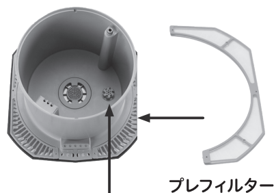
本体ベース
